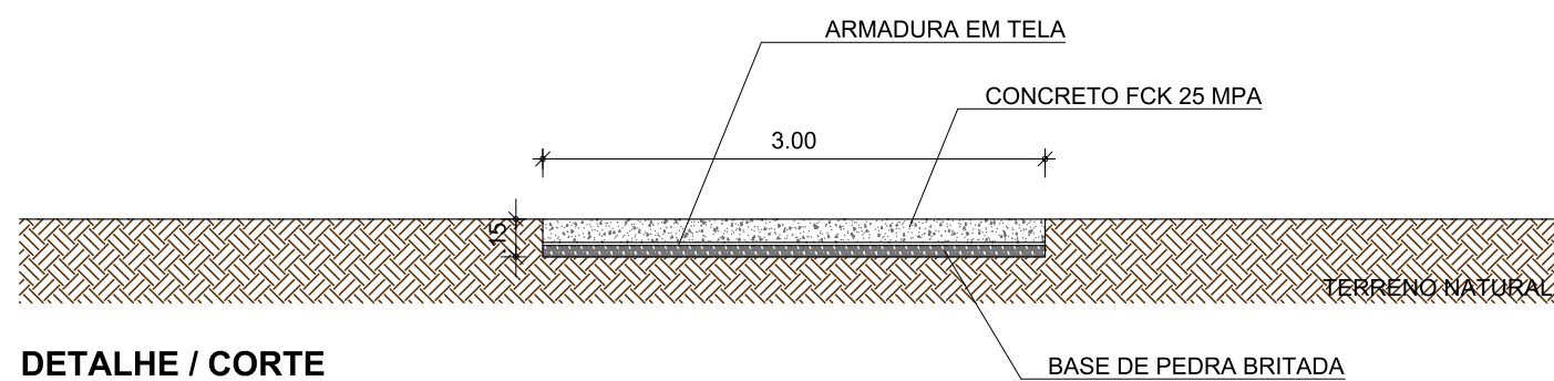
DETALHE / CORTE BASE EM CONCRETO PARA INSTALAÇÃO DE EQUIPAMENTOS Escala 1/50
