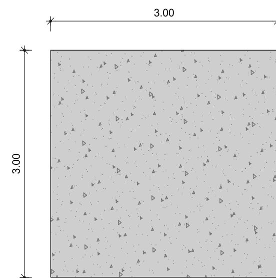
PLANTA BAIXA BASE EM CONCRETO PARA INSTALAÇÃO DE EQUIPAMENTOS Escala 1/50
