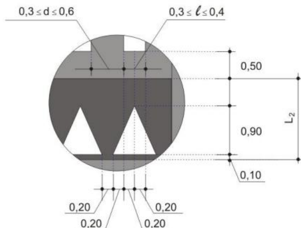
DETALHE A
