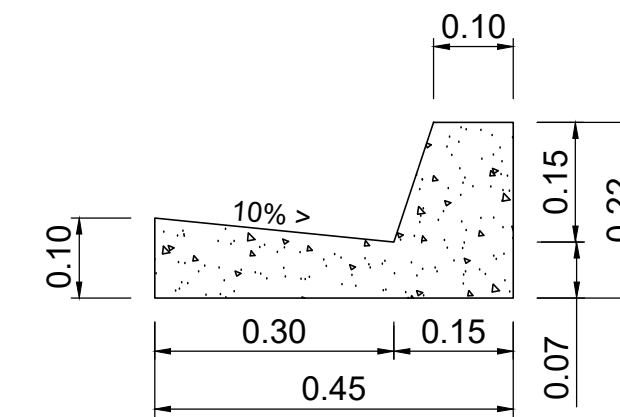
GUIA + SARJETA SEM ESCALA
