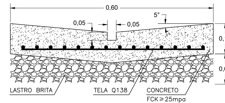
SARJETÃO SEM ESCALA
