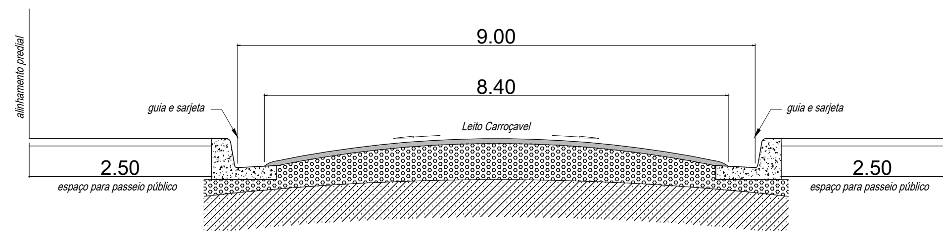
PERFIL TRANSVERSAL DA VIA SEM ESCALA
