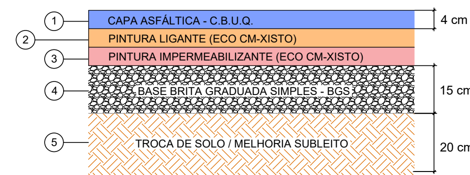
CAMADAS PAVIMENTO SEM ESCALA
